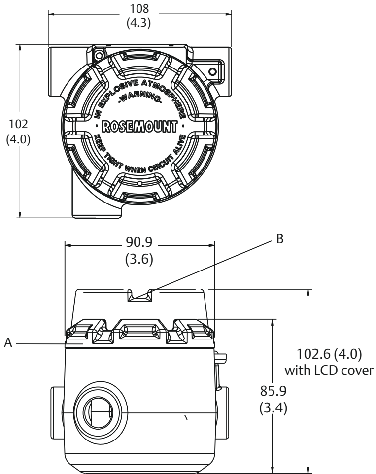
图 9: 螺纹传感器通用连接头, 3 导线管 (选项代码 J1 或 J2)
