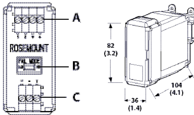
图 5: 罗斯蒙特 644 导轨安装型
