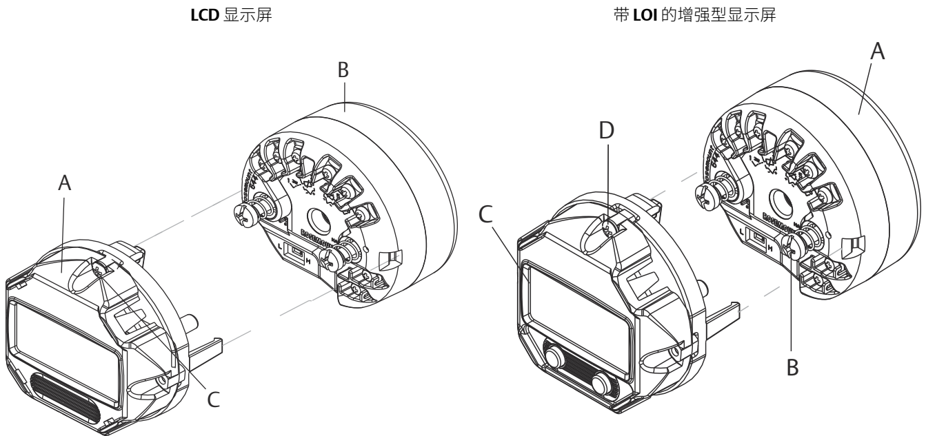
图 12: 显示单元
