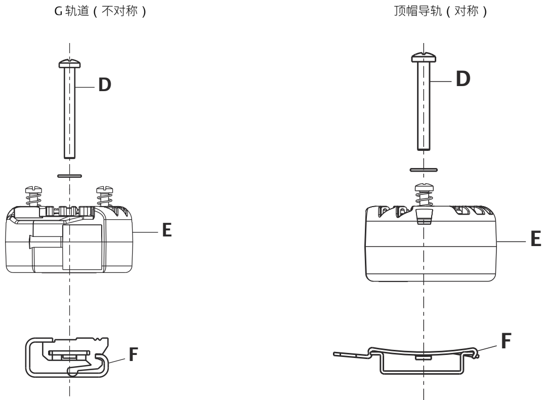
图 7: 罗斯蒙特 644H 导轨夹
