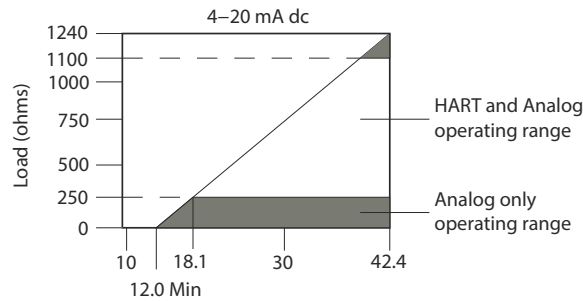
图 2: 负载限制
