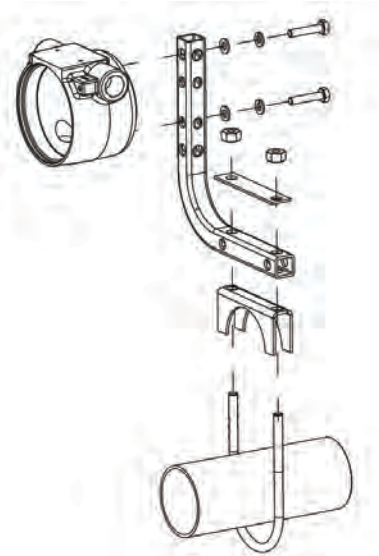
选项代码 B5 用于外壳 J1、J2、J3 和 J4 的支架
