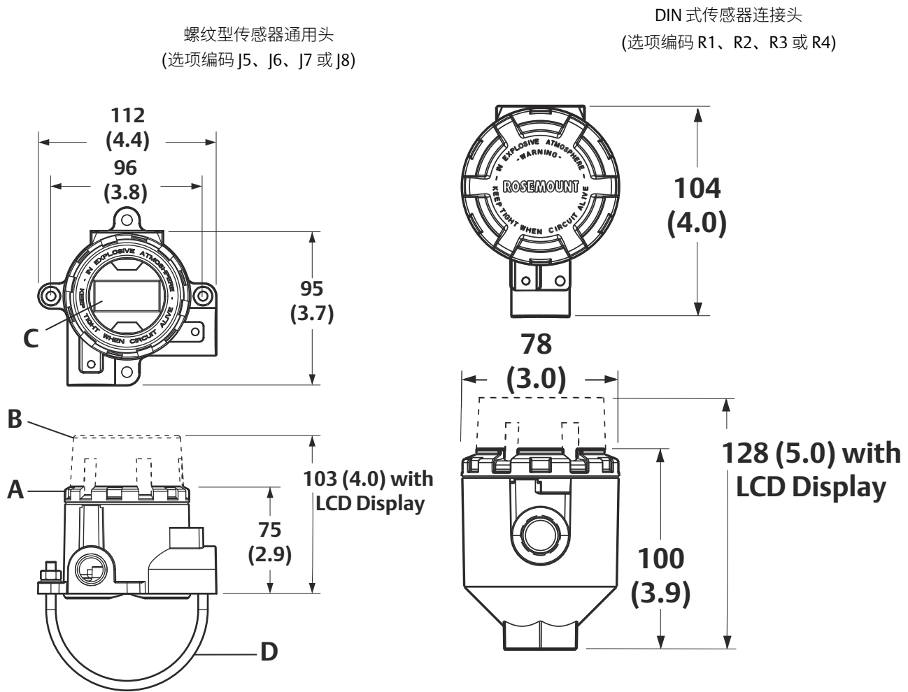
图 8: 螺纹传感器通用连接头和 DIN 式传感器连接头
