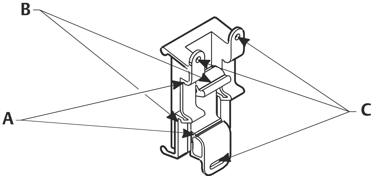
图 6: 罗斯蒙特 644H 的安装套件
